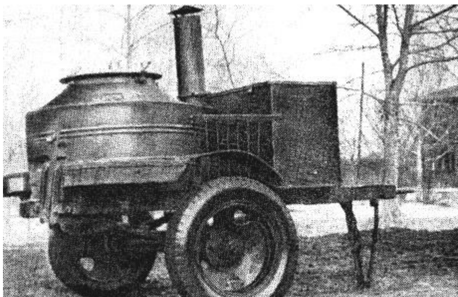
Модель походной кухни КП-42. Фото музея Ирбитского автоагрегатного завода 1940-х гг.
